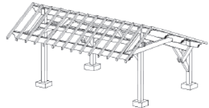
Axonométrie carport 2 places
